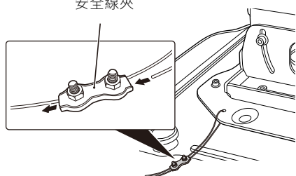
安全線夾
